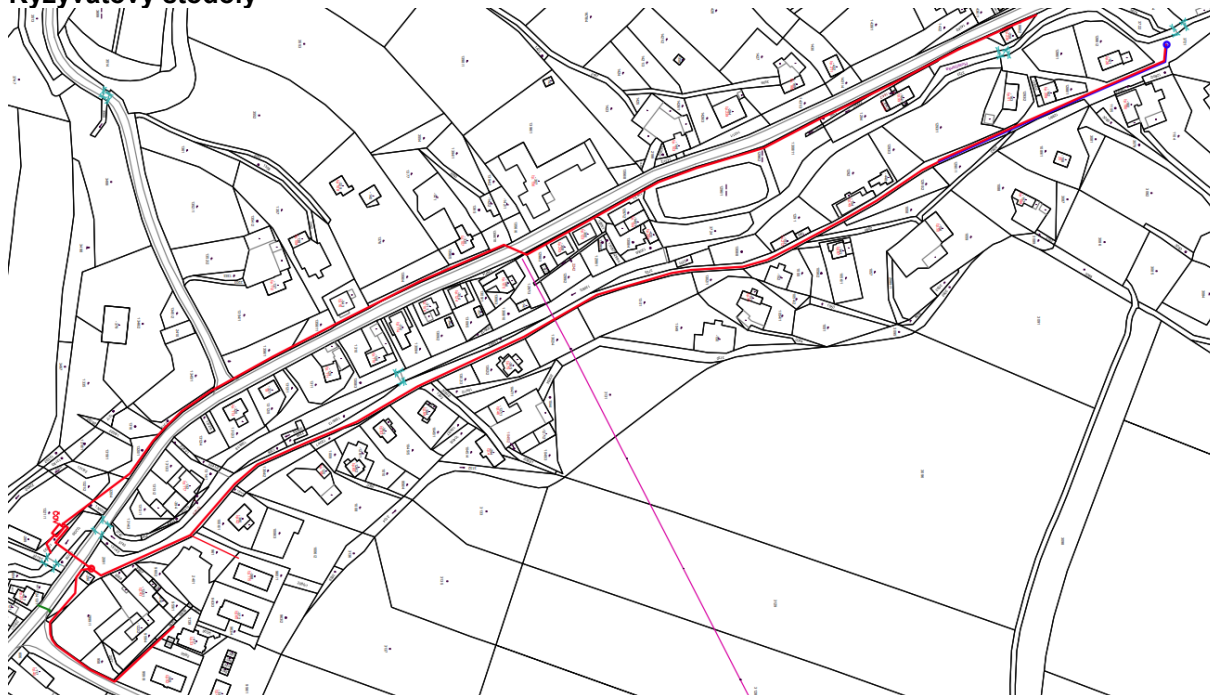
Obrázek 1: Mapka území s dvěma stokami a přečerpávací stanicí u staré hasičárny a ČOV u Kyzvátovy stodoly
